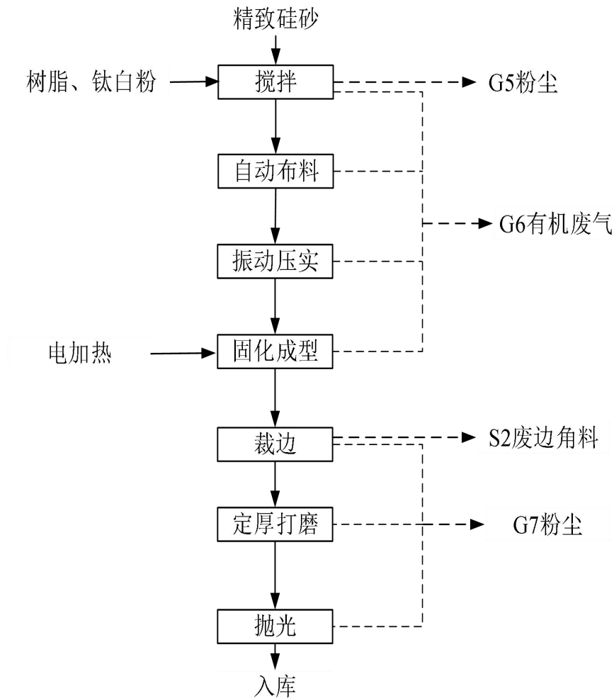
图 3.6-2 项目硅砂板材生产工艺流程及产污环节图
